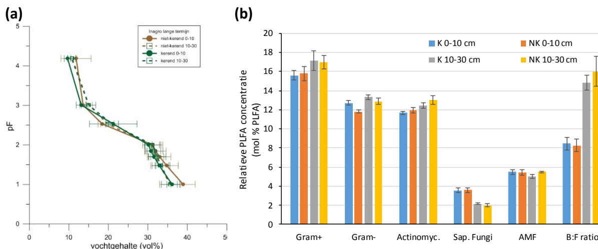
Figuur 24 (a) pF-curve en (b) relatieve PLFA-concentratie in de lange termijnproef bij Inagro.
