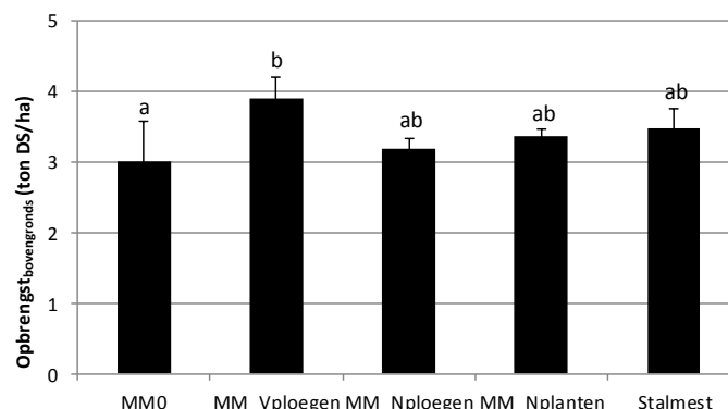
Figuur 18 Bovengrondse droge gewasopbrengst bij tussentijdse staalname (23/07/2015) in de korte termijnproef bij Inagro in 2015 (Gemiddelde en standaarddeviatie, n = 4). Behandelingen met verschillende letters verschillen significant ( P < 0.05 ) volgens een Scheffé-test.
