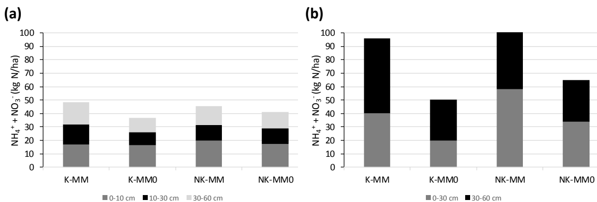
Figuur 27 Bodem minerale N ( \text{NH}_4^+ -N en \text{NO}_3^- -N) concentraties (a) bij aanvang (11/04/2016) en (b) op het einde van de teelt (21/09/2016) in de lange termijnproef bij Inagro in 2016.
